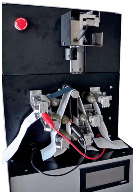
町内企業との連携で製作した電池の安全性を商品化前に判断できる装置（試作機）
